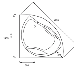
Presqu'île - Corner bath
